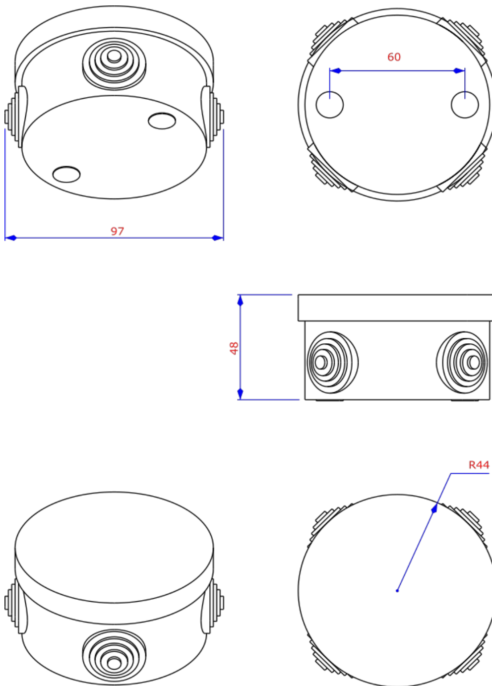
Рис. 2. Габаритные и установочные размеры ПР-3 IP55.
